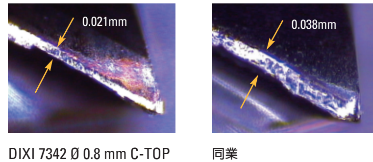
加工47分鐘後的磨損情形
