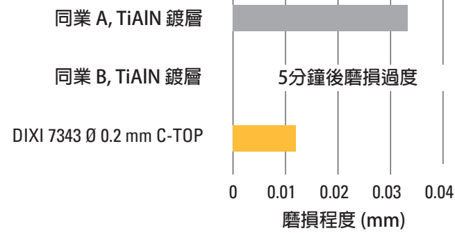
加工51m長度後磨損情形
