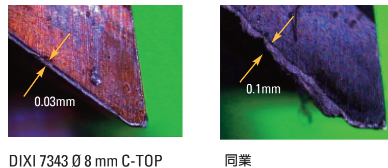
加工16m長度後磨損情形
